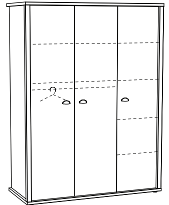
K3 150 x 200 x 64 cm
