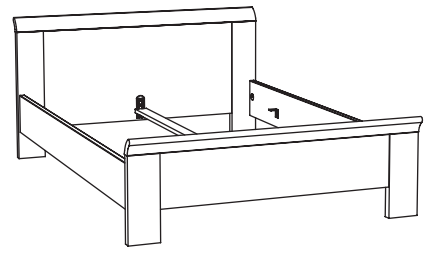
B14 149 x 82 x 215 cm B16 169 x 82 x 215 cm B18 189 x 82 x 215 cm
